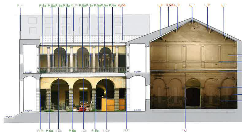
SEZIONE C-C
