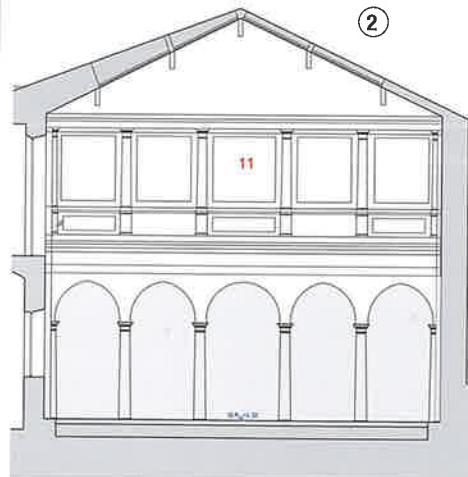
Sezione trasversale, parete ovest
