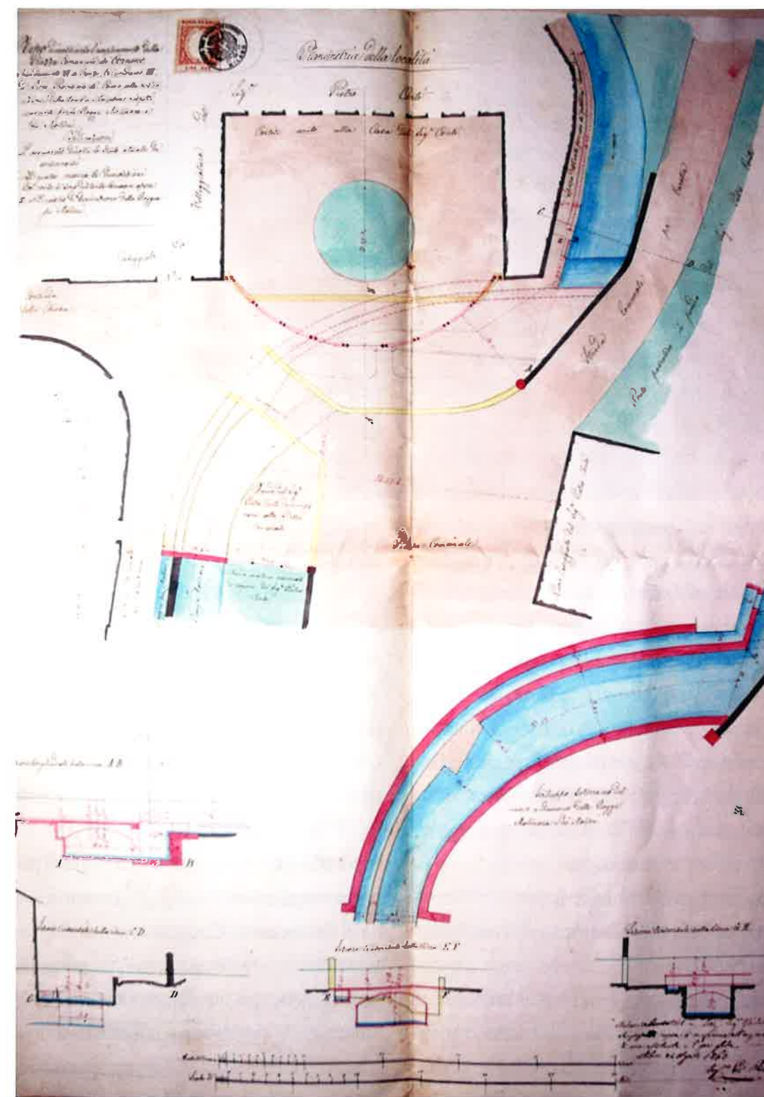
Progettazione delle opere idrauliche per la nuova piazza di Corneno (1863).
