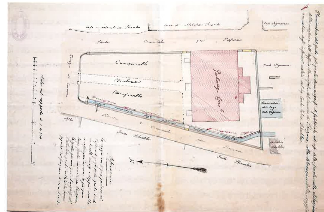
Progettazione del nuovo edificio comunale e scolastico sulla piazza di Corneno.
