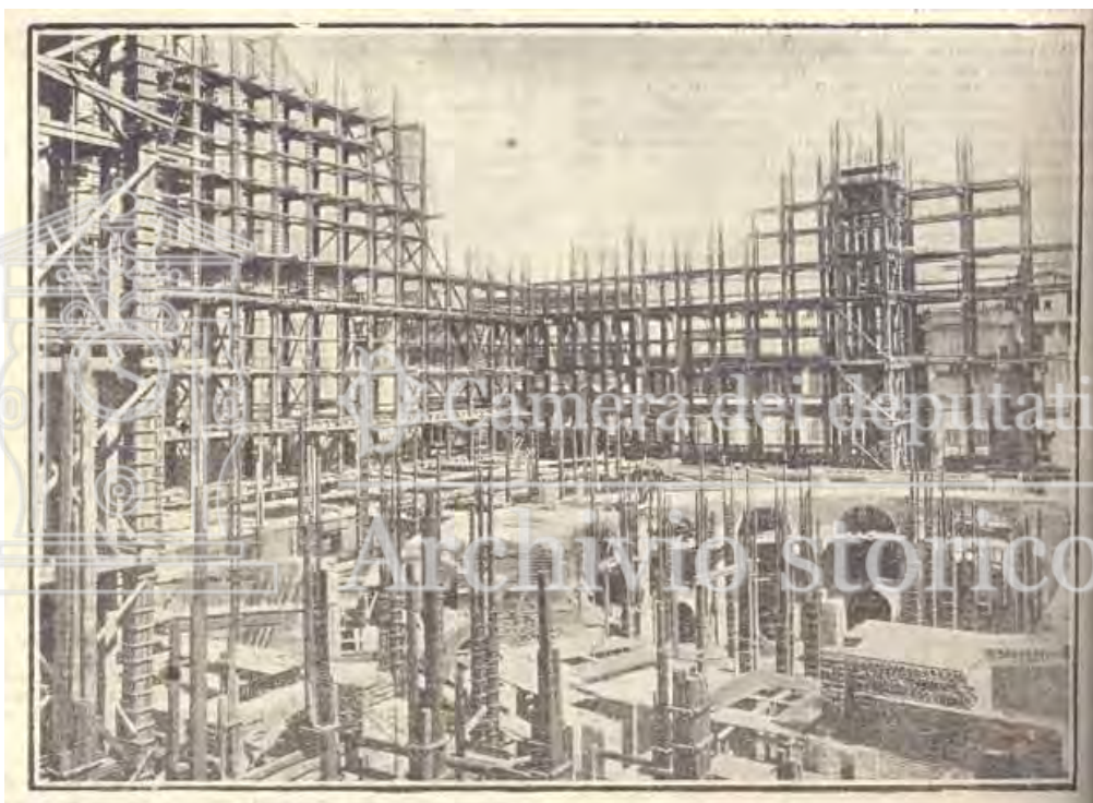
Fondamenta della nuova aula e strutture portanti della facciata ( Tribuna illustrata , 1910)
