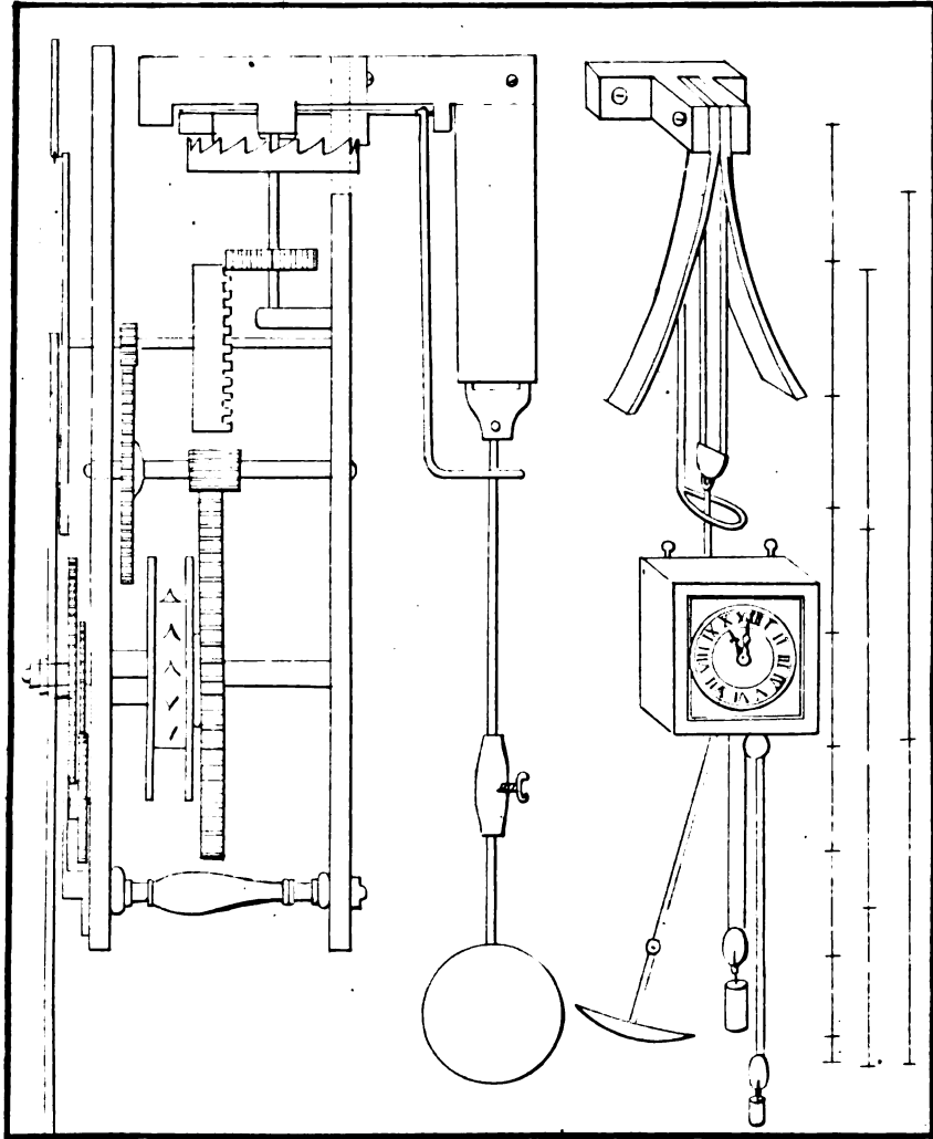
Orologio oscillatorio
