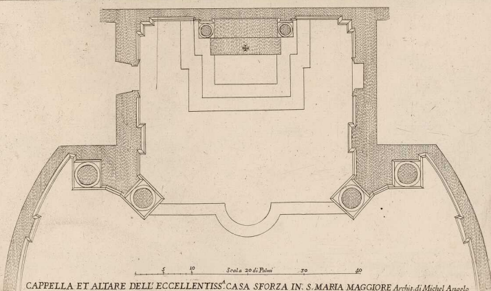
CAPPELLA ET ALTARE DELL' ECCELLENTISS MA CASA SFORZA IN S. MARIA MAGGIORE Archit. di Michel Angelo
