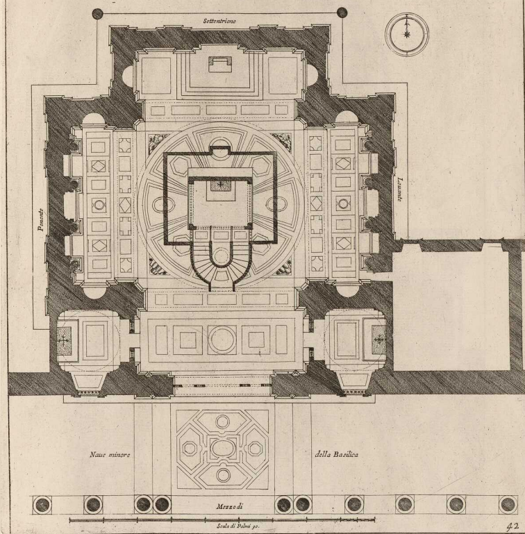
PIANTA DELLA CAPPELLA DEL SANTISSIMO PRESEPE IN SANTA MARIA MAGGIORE EDIFICATA DA SISTO V. Architet o del Cav. Domenico Fontana
