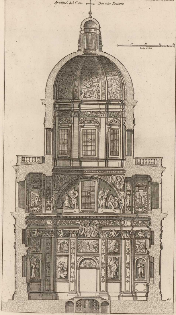
FACCIA INTERIORE PRINCIPALE DELLA CAPPELLA DEL SANTISSIMO PRESEPE DI NOSTRO SIGNORE NELLA BASILICA LIBERIANA DI SANTA MARIA MAGGIORE DA SISTO V CON PONTIFICIA MVNIFICENZA EDIFICATA Architet. del Cav. Domenico Fontana
