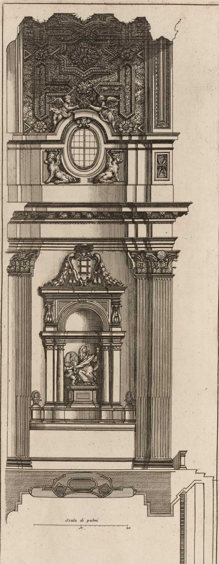
FIANCO DELL' ALTARE MAGGIORE DELLA CHIESA DI SAN GIOVANNI DE FIORENTINI CON LI DEPOSITI DE SIGNORI FALCONIERI Architettura del Cau. Borromini sino alli capitelli delli sudetti Depositi. La parte superiore di Ciro Ferri.
