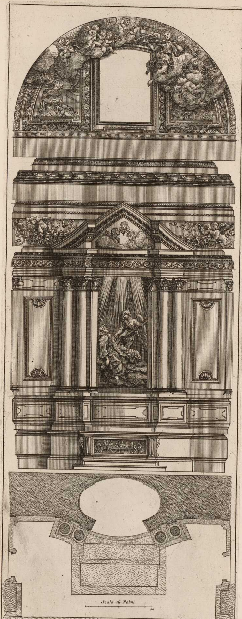
CAPPELLA, E ALTARE DE SIGNORI CORNARI NELLA CHIESA DELLA MADONNA DELLA VITTORIA Disegnato da Gio. Innocenzo Rizzi in Roma, alla Architettura del Cav. Bernini. Vin. Marconi Sculp. 21
