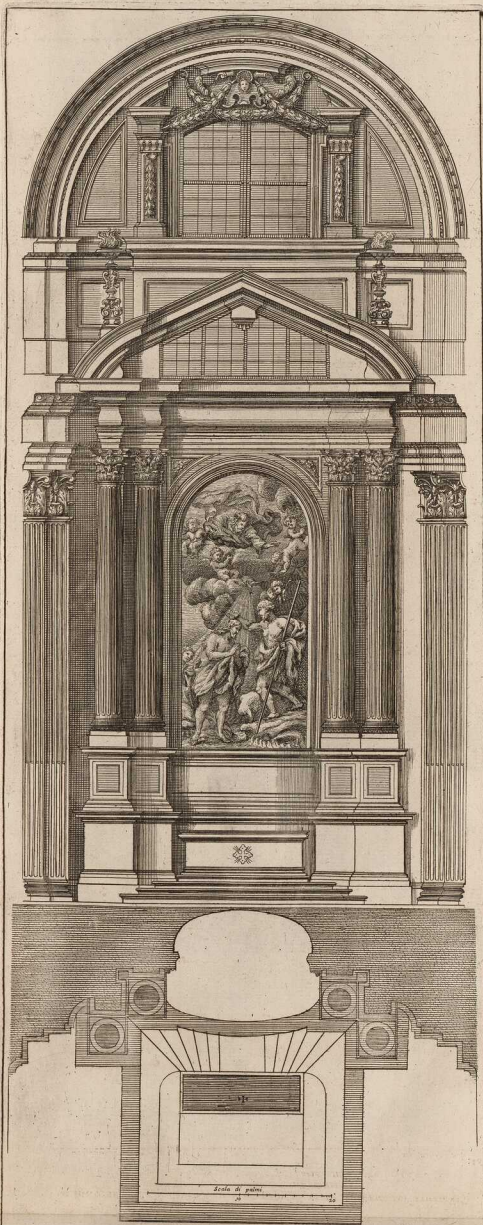
ALTARE MAGGIORE NELLA CHIESA DI SAN GIOVANNI DE FIORENTINI EDIFICATO ET ORNATO DA SIGNORI FALCONERI. Architettura del Cau. Borromeo sino al cornicione, la parte superiore di Ciro Ferri.
