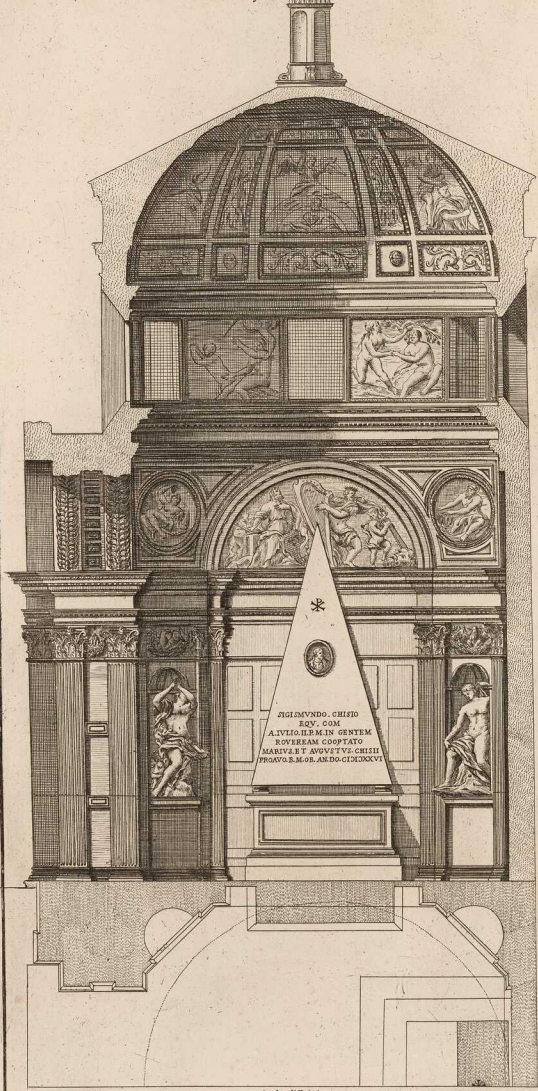
FIANCO DELLA CAPPELLA DELL' ECC. MA CASA CHIGI NELLA CHIESA DI S. MARIA DEL POPOLO Archit. di Raffaele da Urbino
