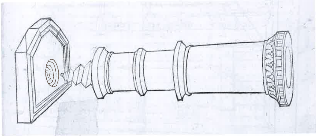
INVENTUM est quoque alterum Machinae huiusce tuum Sigismonde Pandulfe: Qua pilae aeneae tormentarii pulveris plenae cum fungi aridi fomte urientis emittuntur.
