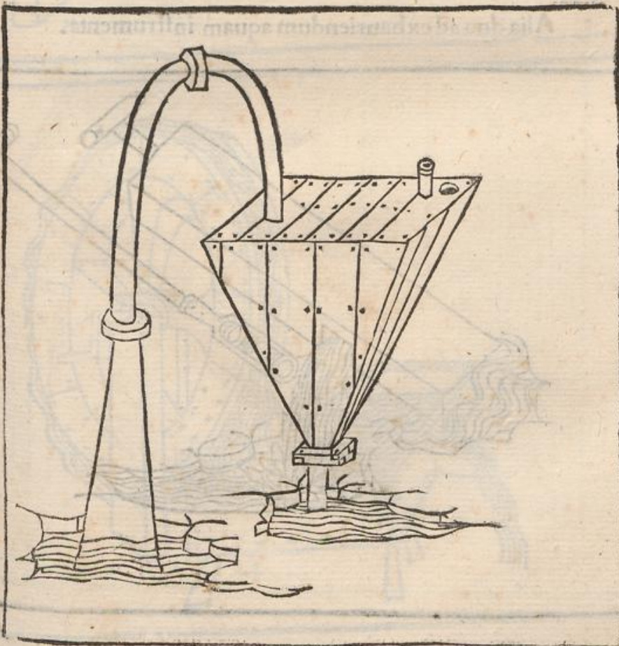
Aliud educendi aquam instrumentum
