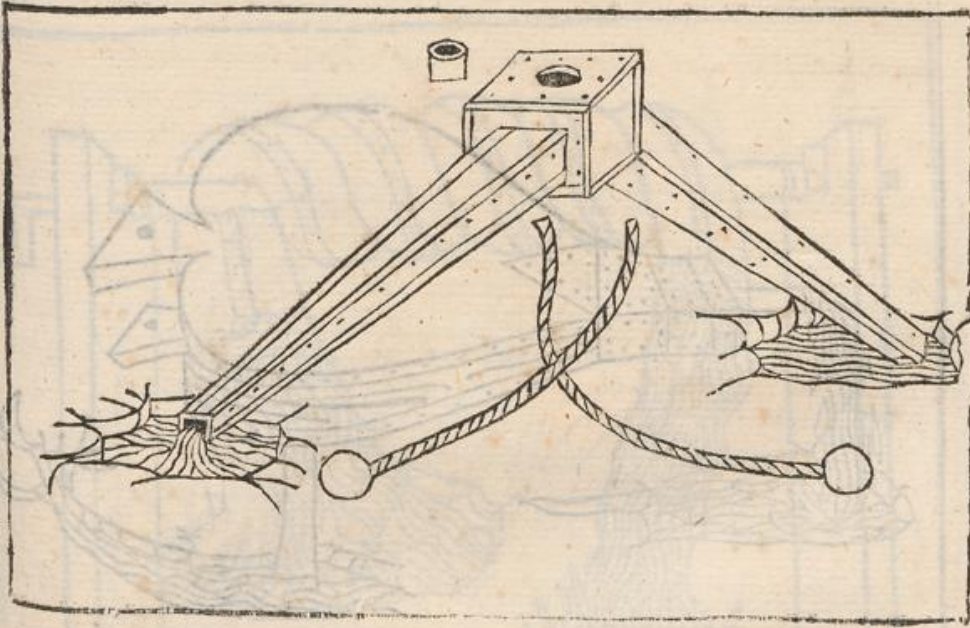
Aliud educendi aquam instrumentum
